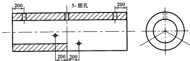
图 1 综合性能测试用对比试样示意图
